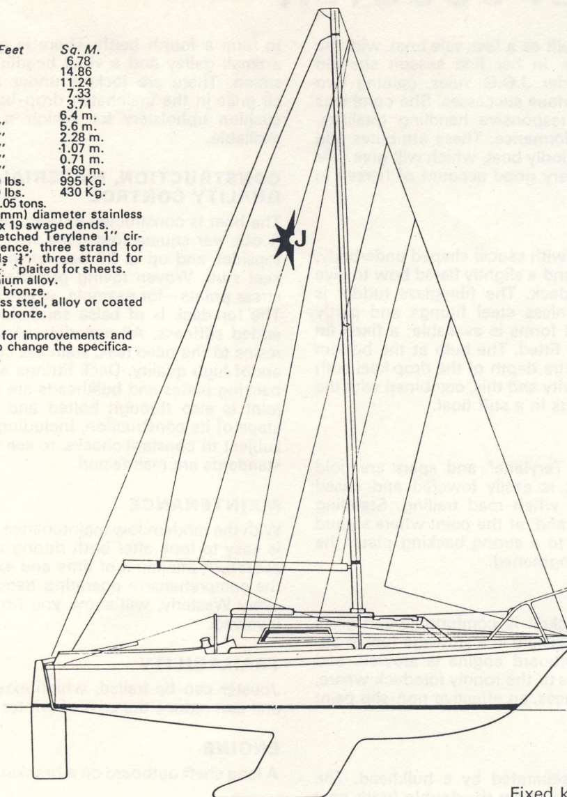
Fixed keel version
